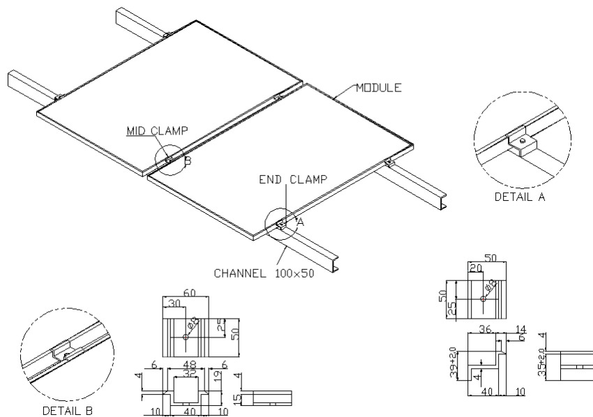
그림 4. 클램핑 방식 설치 방법
