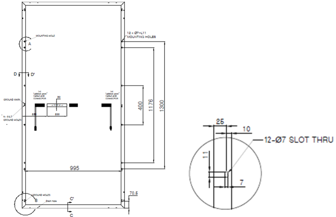
그림 1. 모듈 볼팅 홀 위치 (예시)
