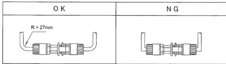
그림 7. Cable Routing
