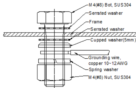
그림 5. Grounding Hardware
