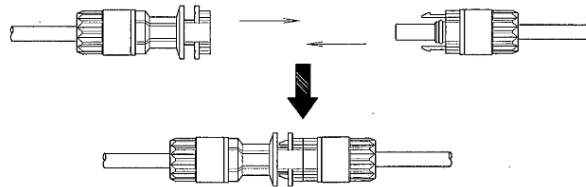
그림 8. Connect connectors
