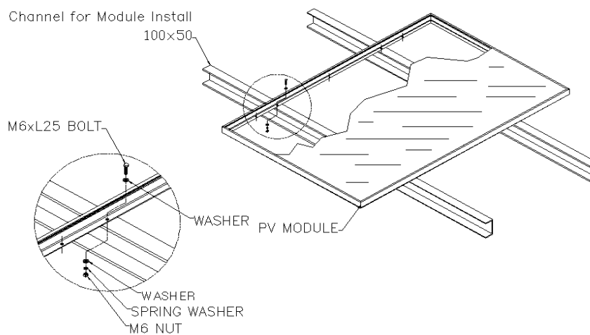
그림 2. 볼팅 방식 설치 방법
