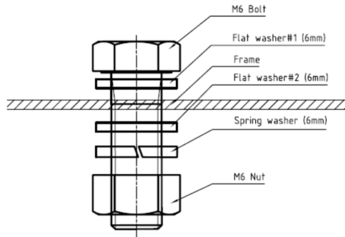
그림 3. 볼팅 방식 부품 (M6 예시)
