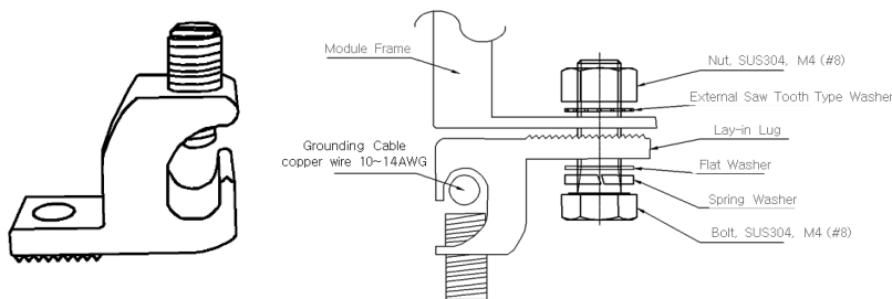
그림 6. Lay in Ground Lug
